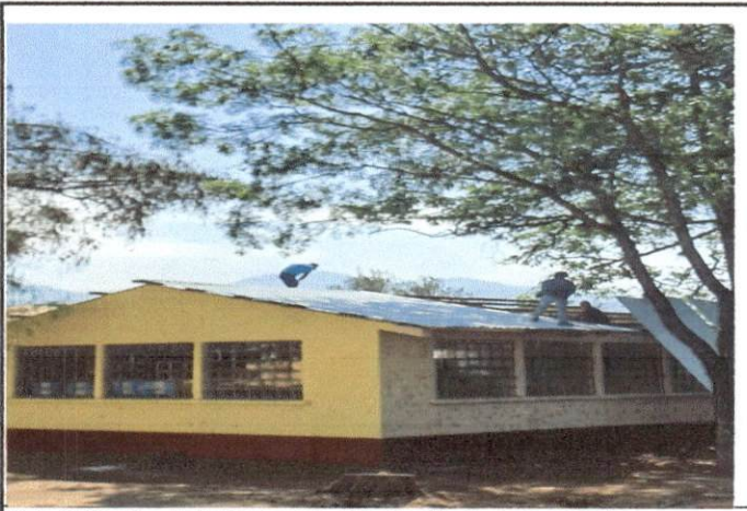
Foto 4: Cambio de techo en aula ubicada al este de la escuela.
